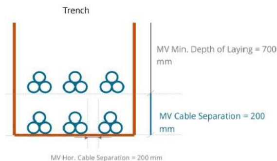
Figura 8. Sección transversal simplificada de una zanja MT.
